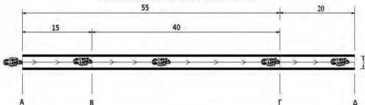
ΣΧΕΔΙΟ 2 ΑΠΕΙΚΟΝΙΣΗ ΧΩΡΟΥ ΔΟΚΙΜΑΣΙΑΣ ΠΕΔΗΣΗΣ ΕΚΤΑΚΤΟΥ ΑΝΑΓΚΗΣ
